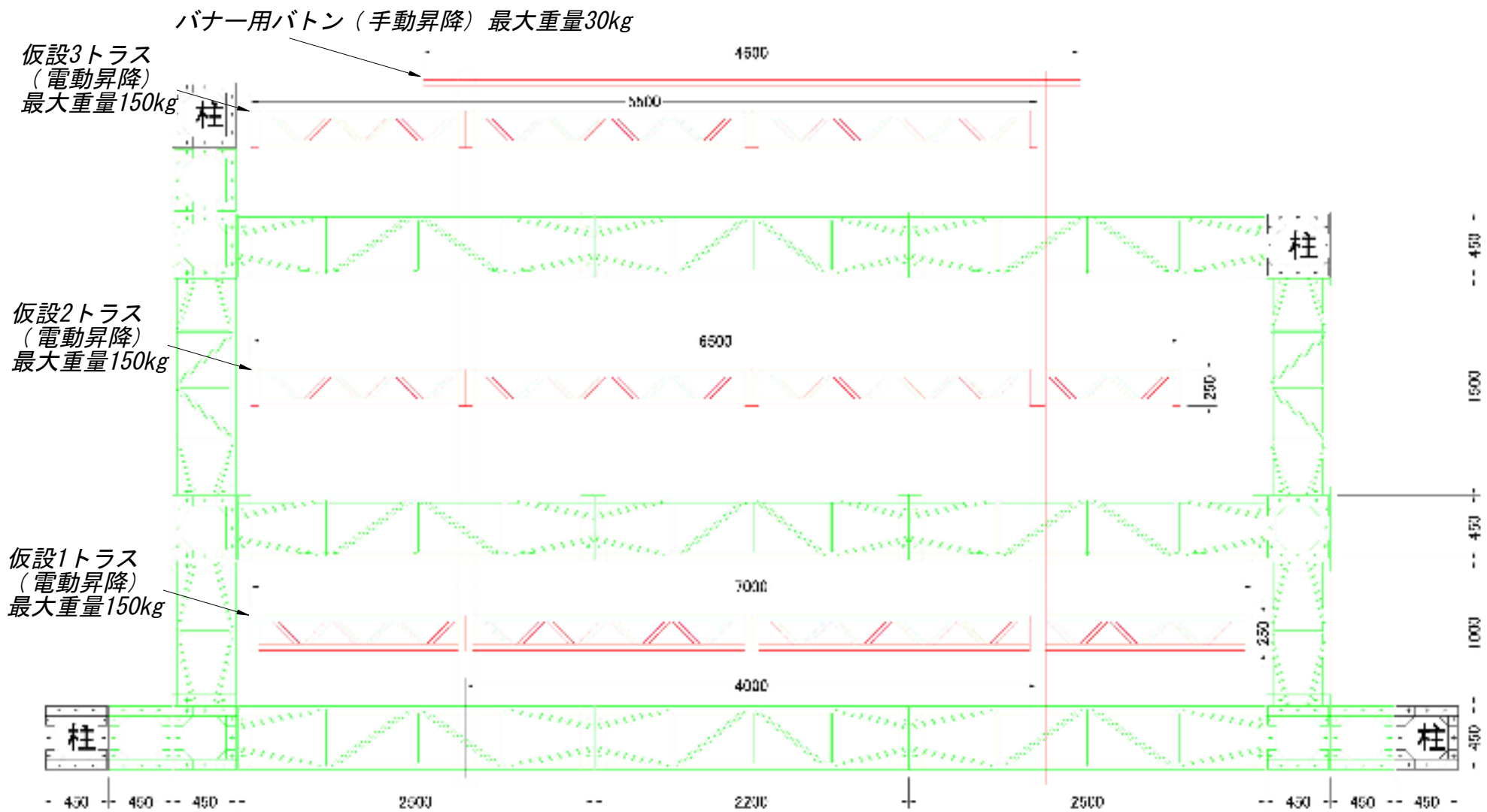
高松festhalle トラス図
